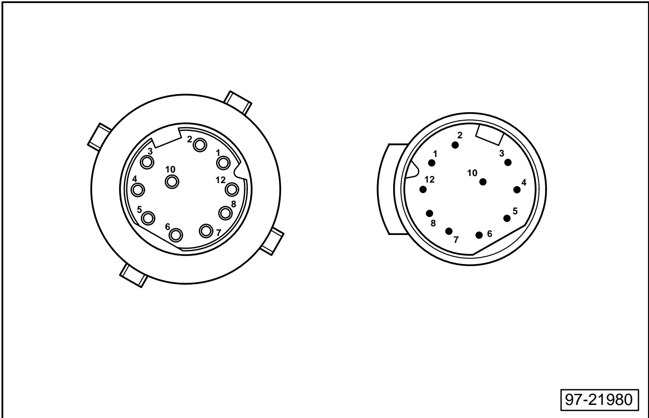
Leitungsstrang
